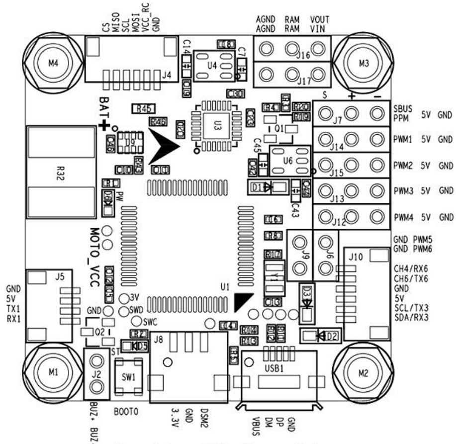
OmnibusF4-Pro-0A
