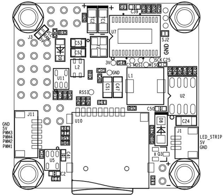
OmnibusF4-Pro-0A
